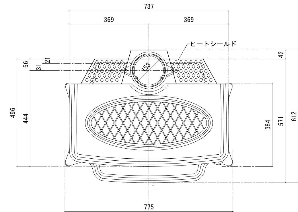
[ 上 面 図 ]
