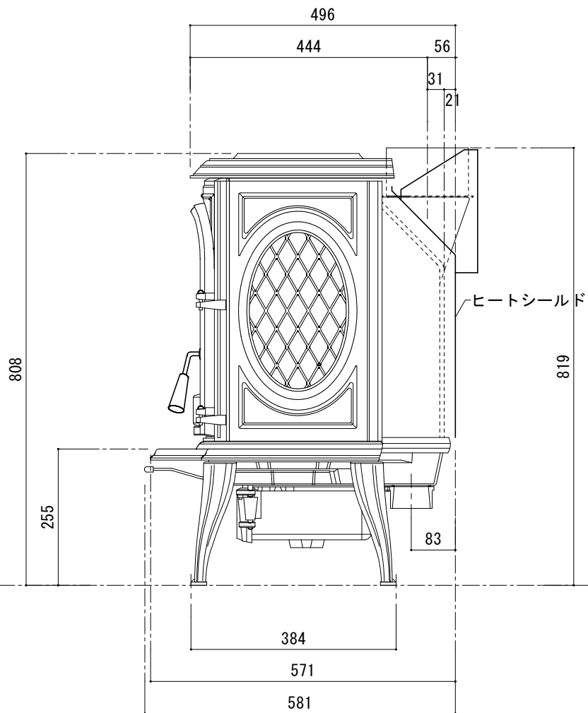
[ 側 面 図 ]
