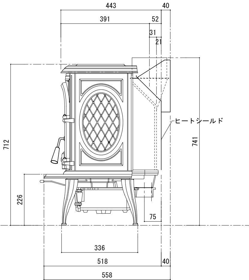
[ 側 面 図 ]
