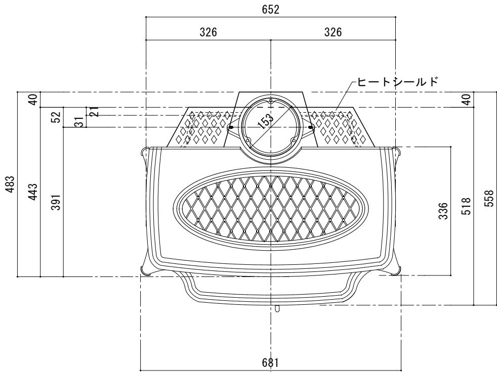
[ 上 面 図 ]
