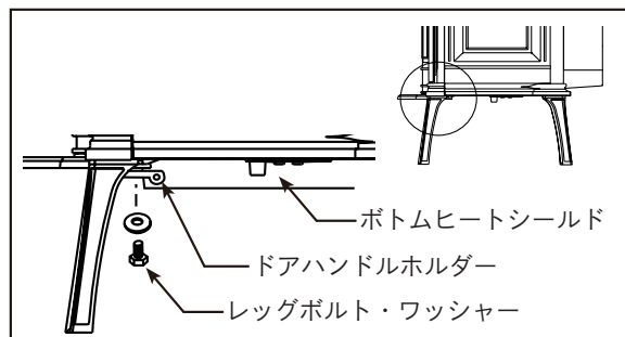
図3 ハンドルホルダーとヒートシールドの位置
