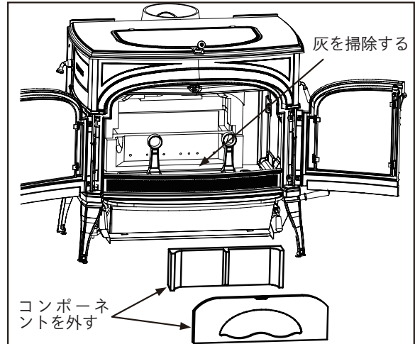
図 27 燃焼システムの背後にたまった灰を点検、掃除します。
