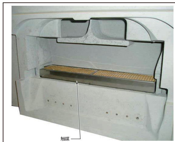
図 12 触媒の取り外し
