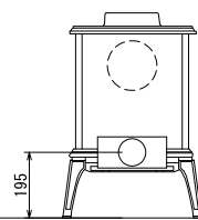
背面図
