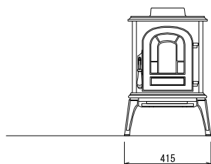
正面図
