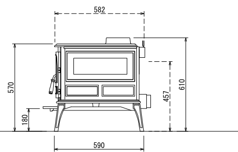
側面図
